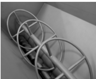
L'agitateur de produit en option empêche toute formation de voûte
